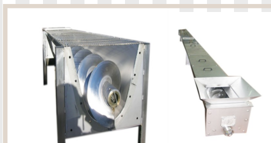
CANALETTE TRASPORTO VINACCIA FERMENTATA/ MACERATO/ESAUSTO E RASPI
